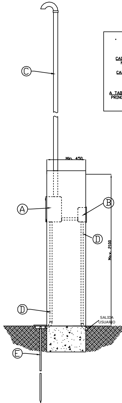
VISTA FRONTAL Caja de Medidor
