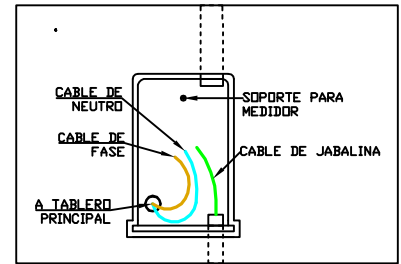
VISTA FRONTAL Caja de Medidor
